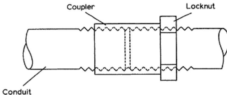
Figure 3.1 Conduit coupling
