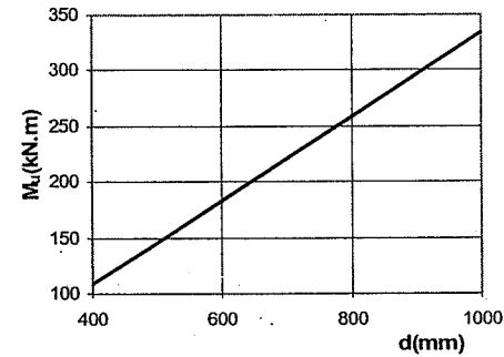
D-Effect of beam depth (d)
