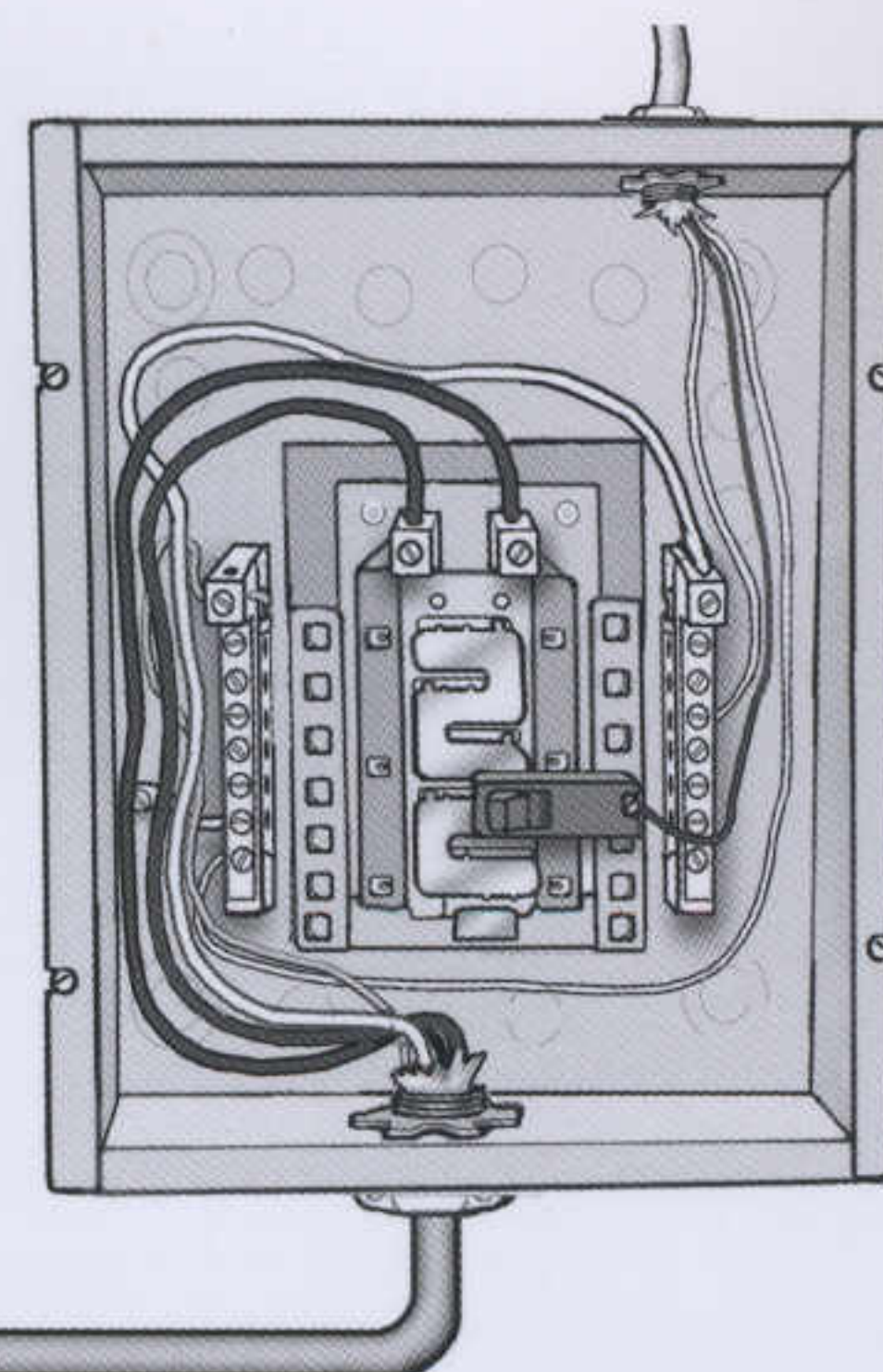
Fig. 32 Subpanel
