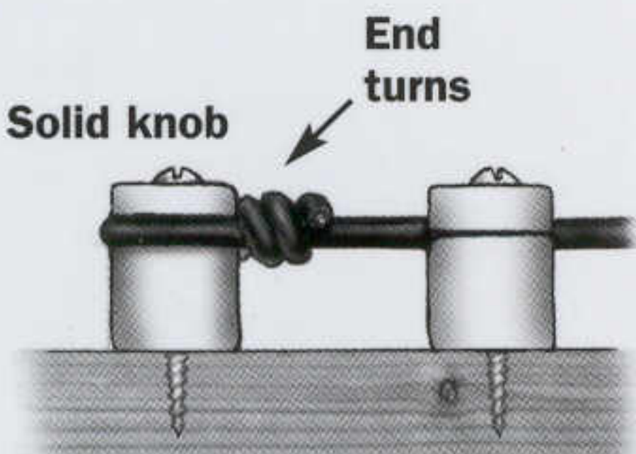
Fig. 89 Splice Wrap
