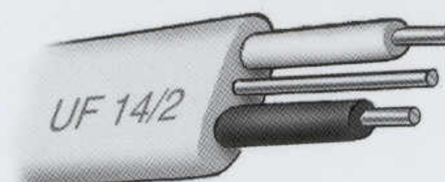
Fig. 47 UF Cable
