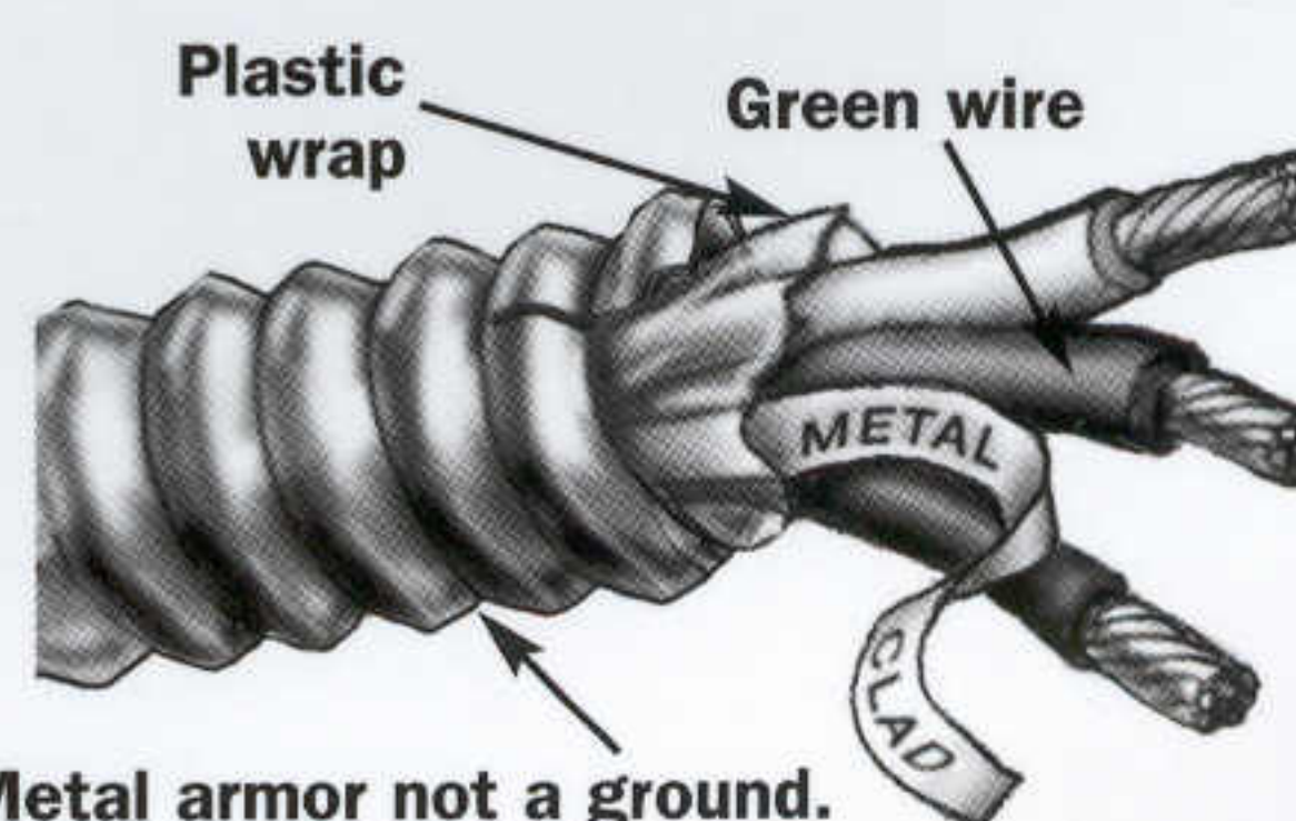
Fig. 49 • MC Cable
